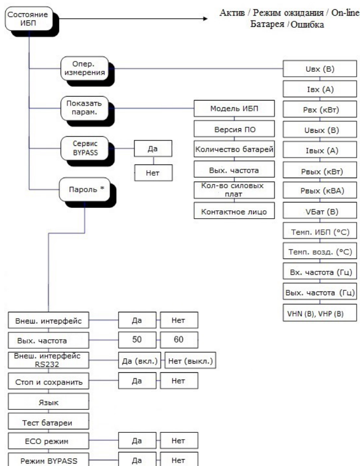
Рисунок 3 – Блок-схема ПО ИБП
