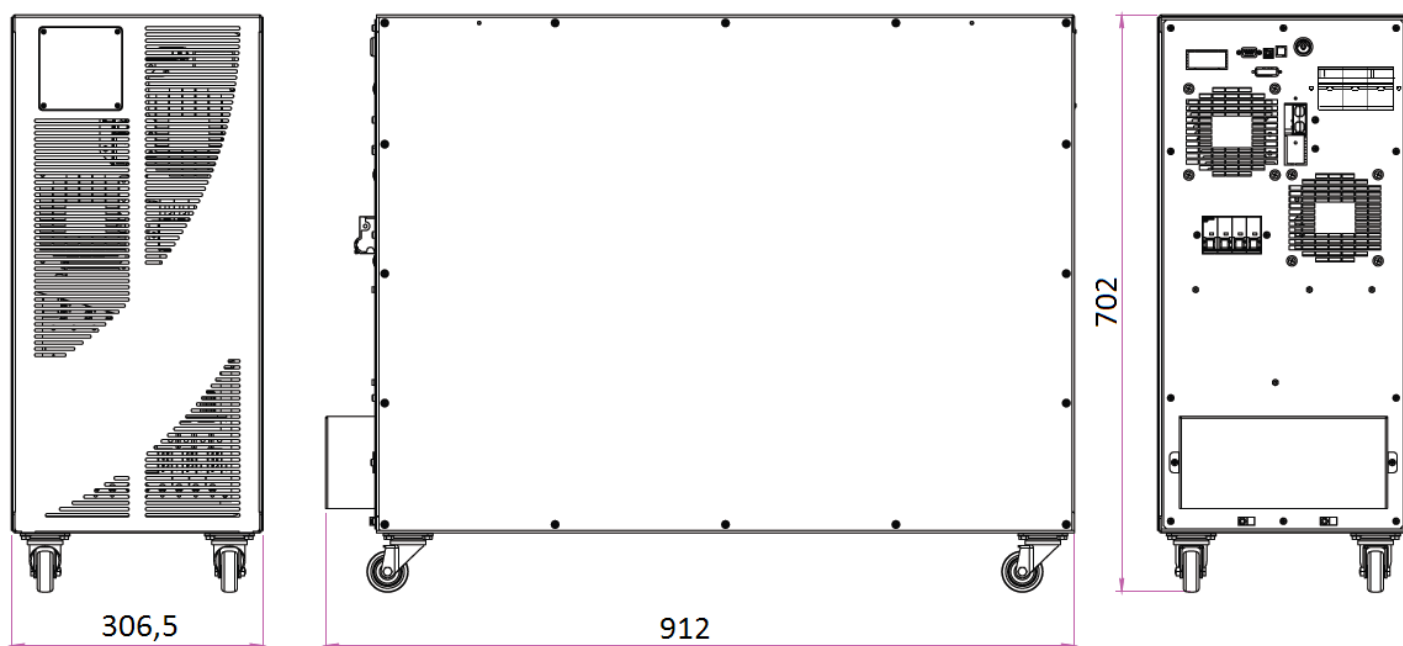
Рисунок 5. Внешний вид ИБП серии Solo MMB
