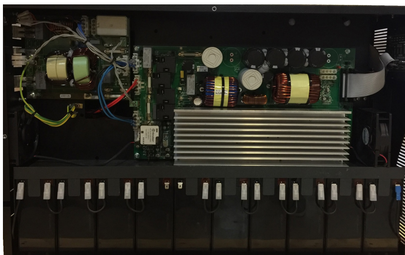
Рисунок 9. Расположение батарей 7/9 Ач Solo MD
