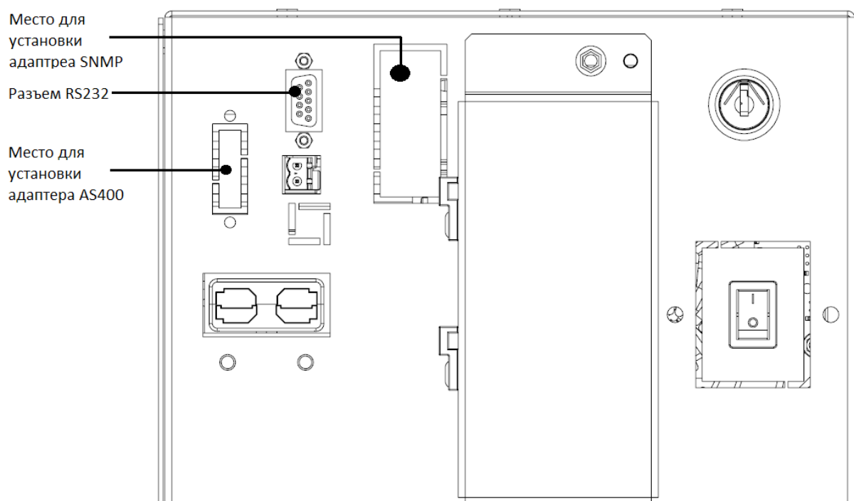
Рисунок 13. Интерфейсы Solo MD
