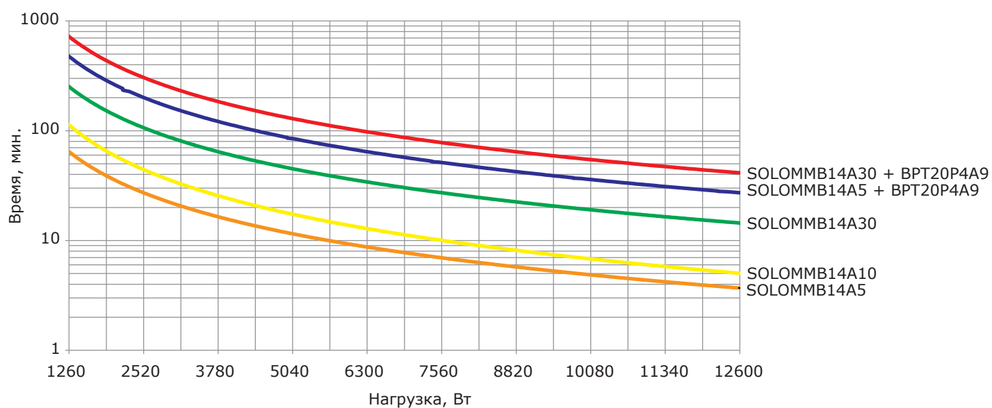
Рисунок 10 – Разрядные характеристики модели SOLOMMB14
