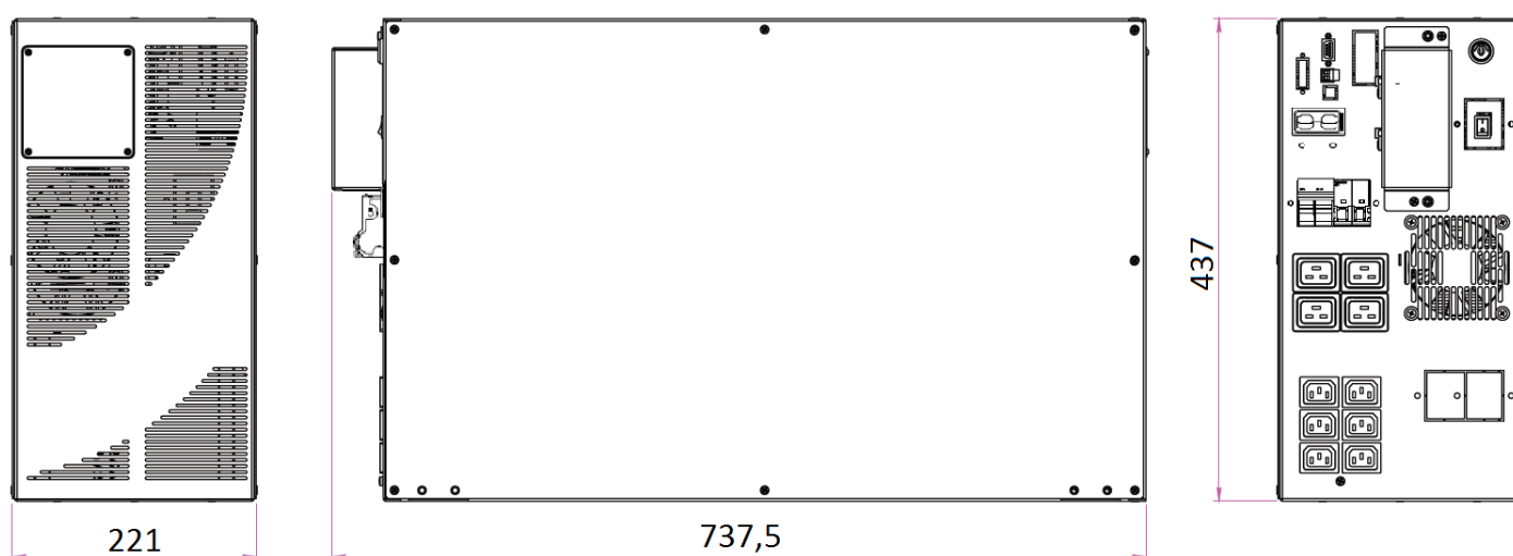
Рисунок 1. Внешний вид ИБП серии Solo MD (вертикальная установка)
