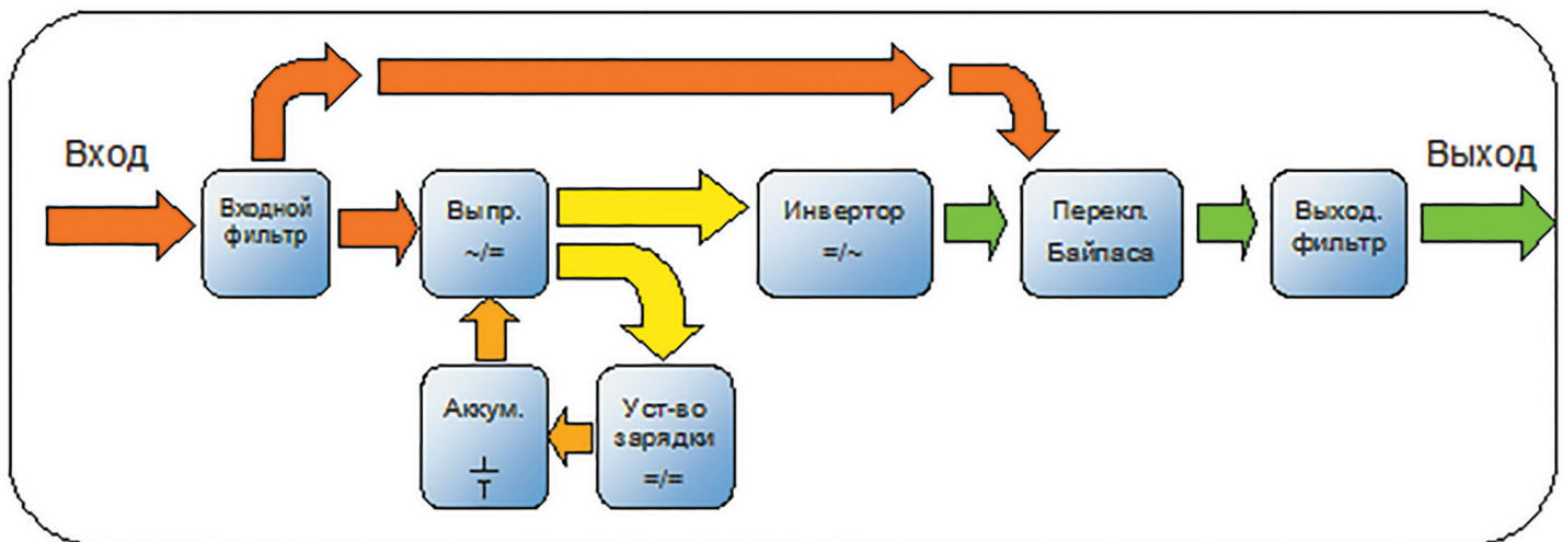
Рисунок 1 – Блок-схема
