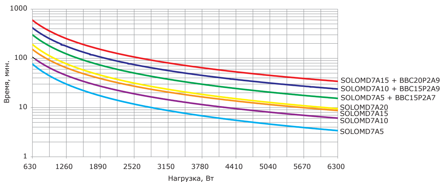
Рисунок 7 – Разрядные характеристики модели SOLOMD7
