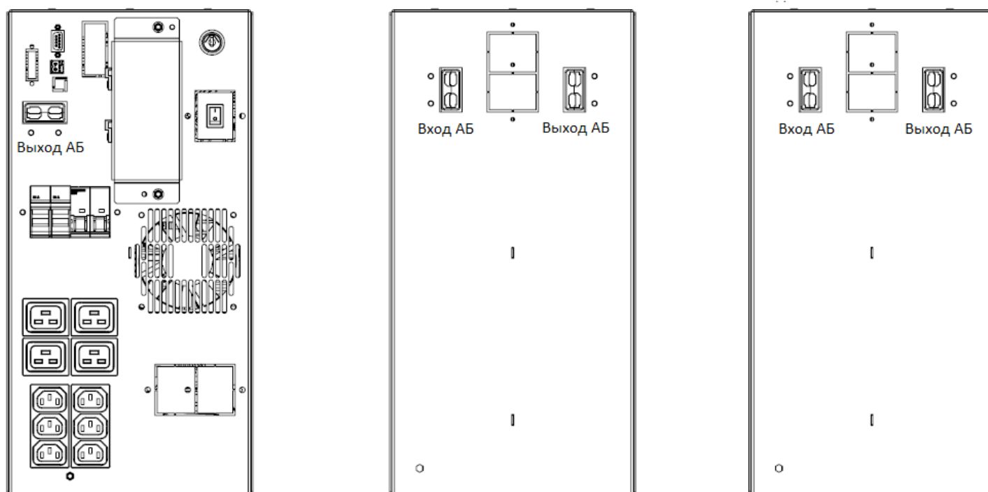
Рисунок 12. Подключение внешних батарейных блоков к ИБП серии Solo MD
