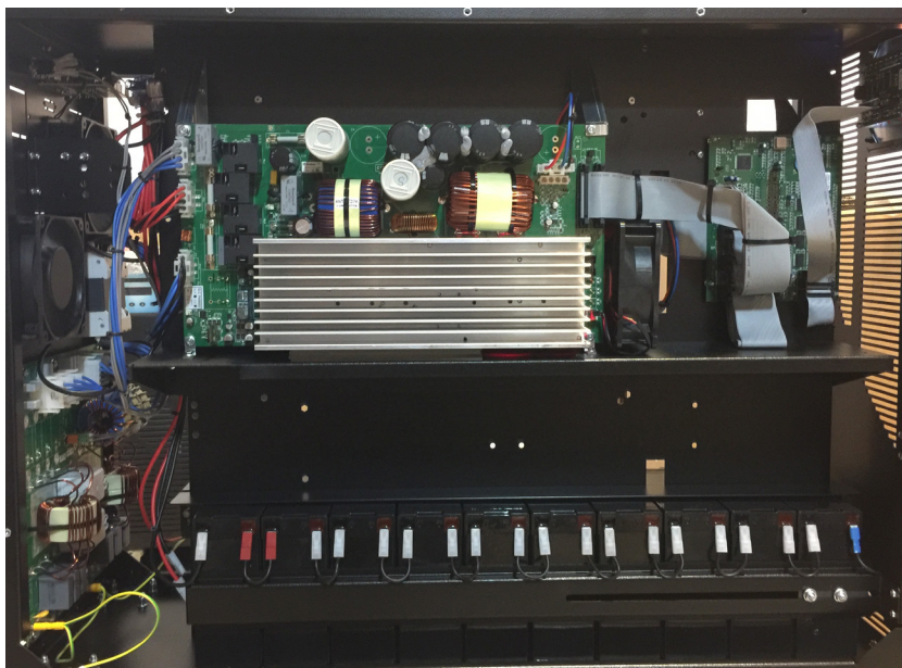
Рисунок 11. Расположение батарей 7Ач,9Ач SOLOMMB 14 кВА
