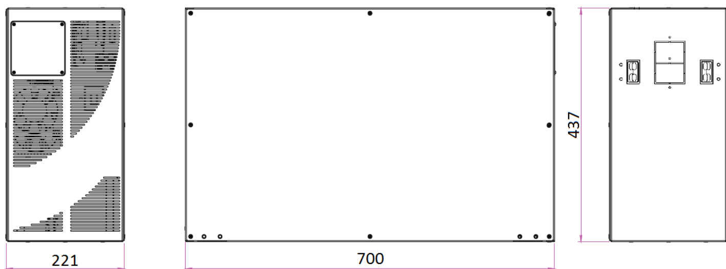
Рисунок 3. Внешний вид батарейного блока серии Solo MD (вертикальная установка)
