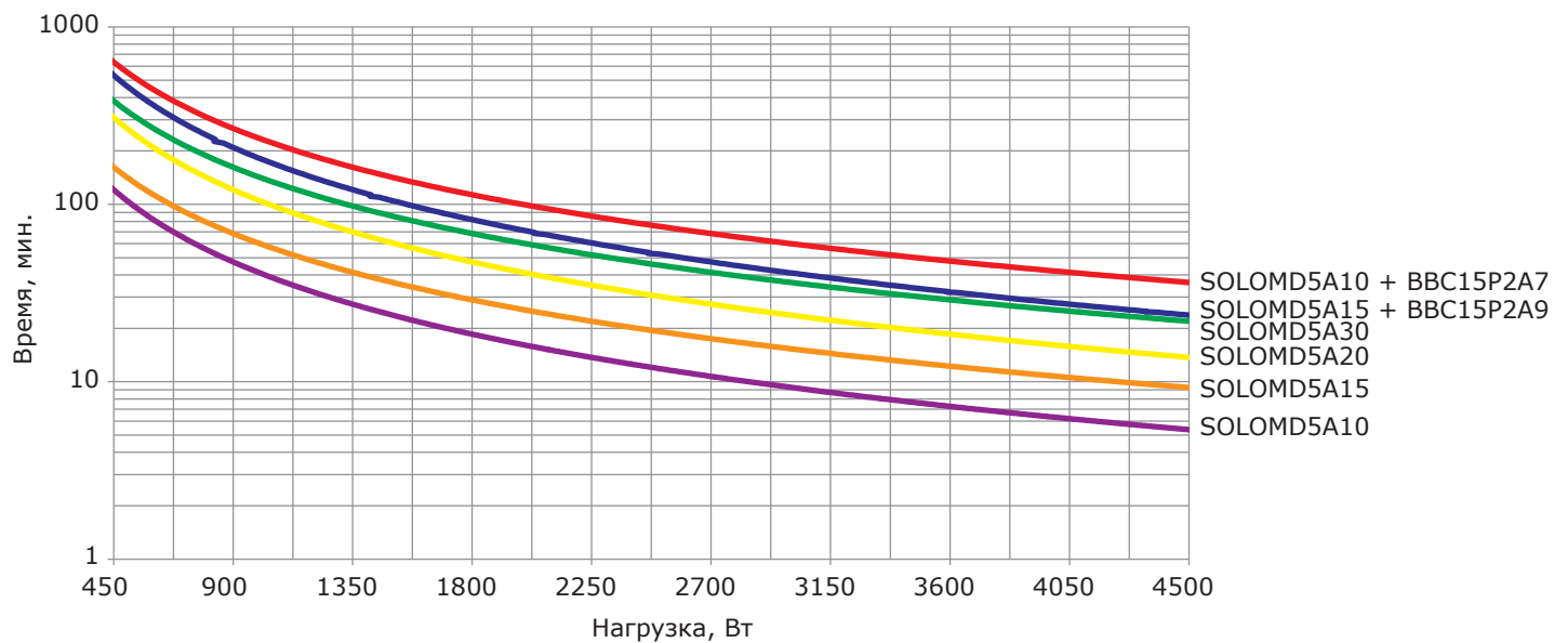
Рисунок 5 – Разрядные характеристики модели SOLOMD5
