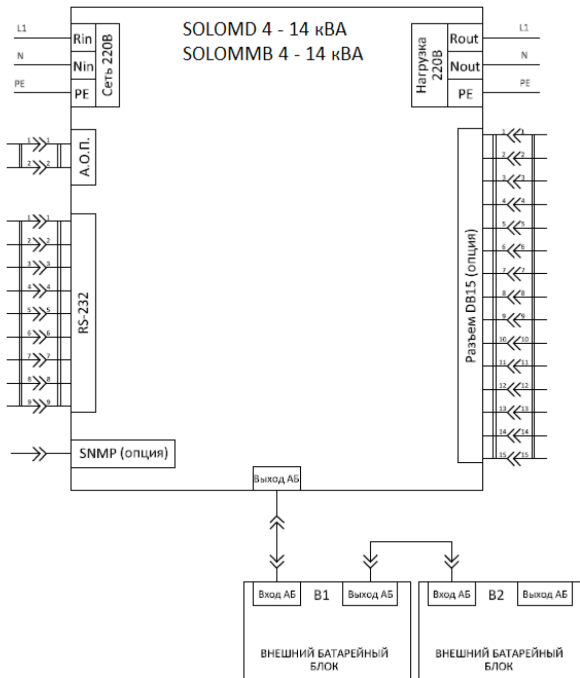
Рисунок 8. Схема подключения ИБП серии Solo
