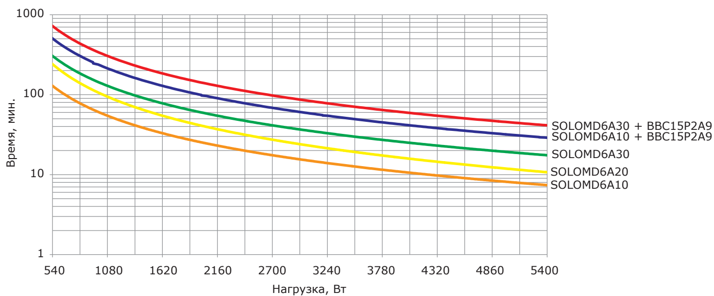
Рисунок 6 – Разрядные характеристики модели SOLOMD6
