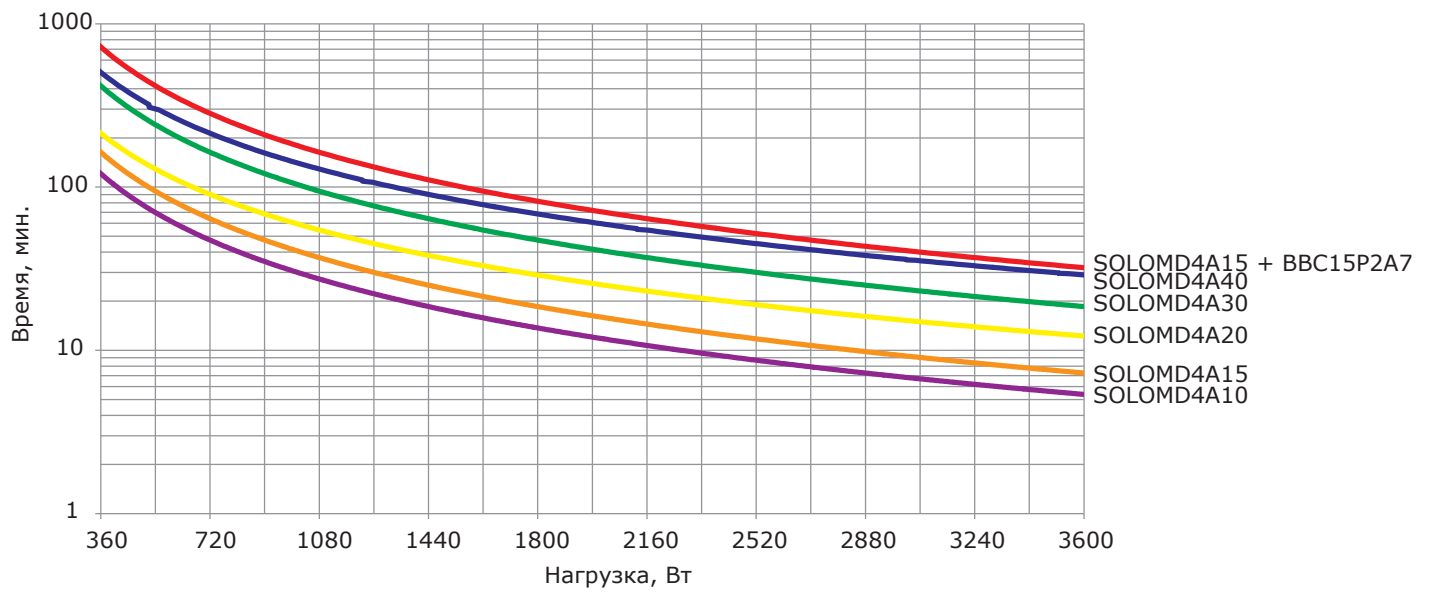
Рисунок 4 – Разрядные характеристики модели SOLOMD4
