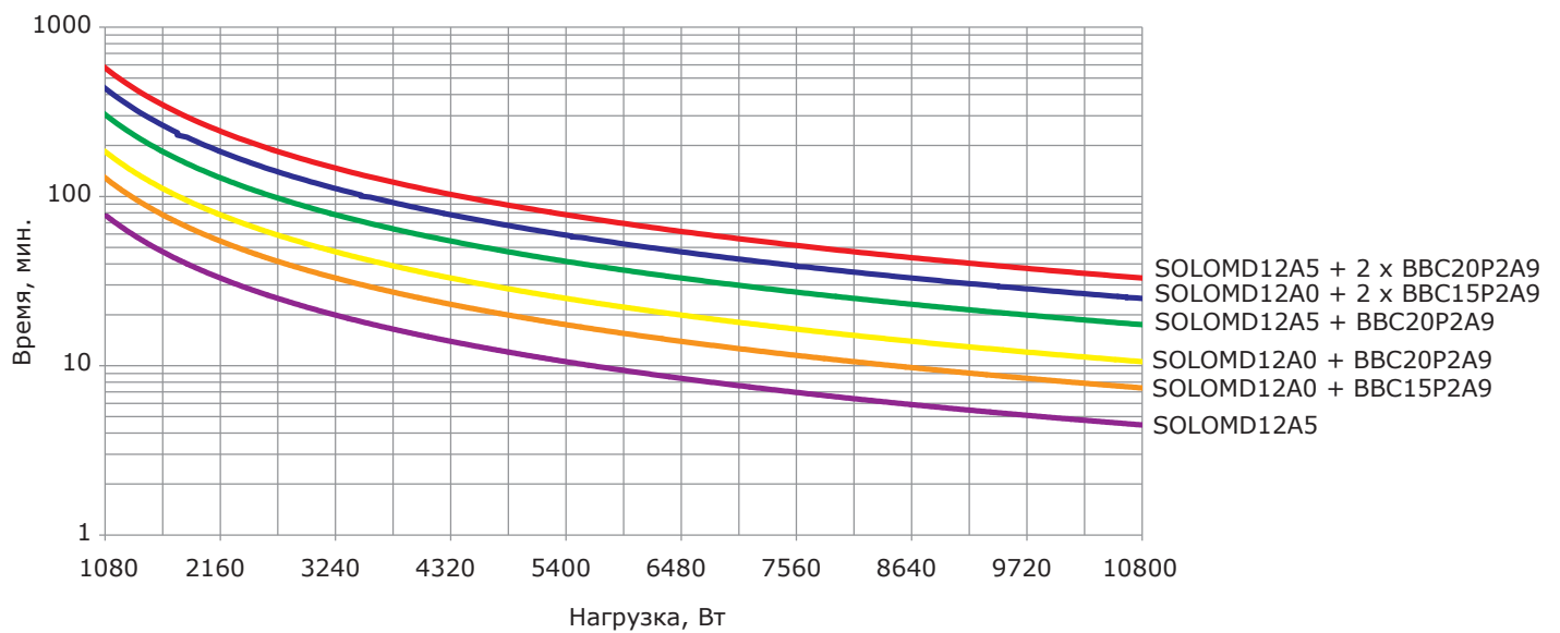
Рисунок 9 – Разрядные характеристики модели SOLOMD12
