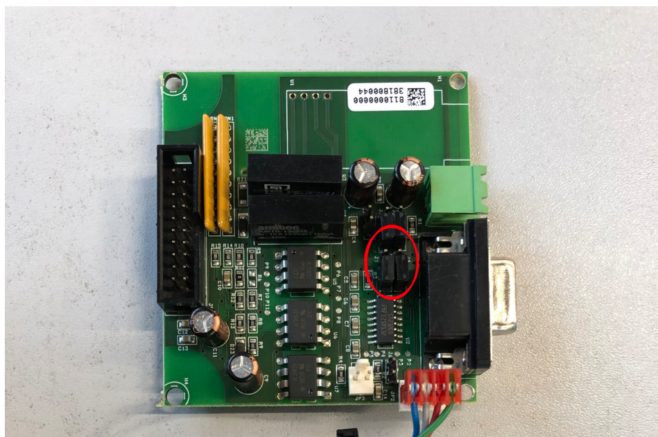
Рисунок 14. Подключение платы SNMP
