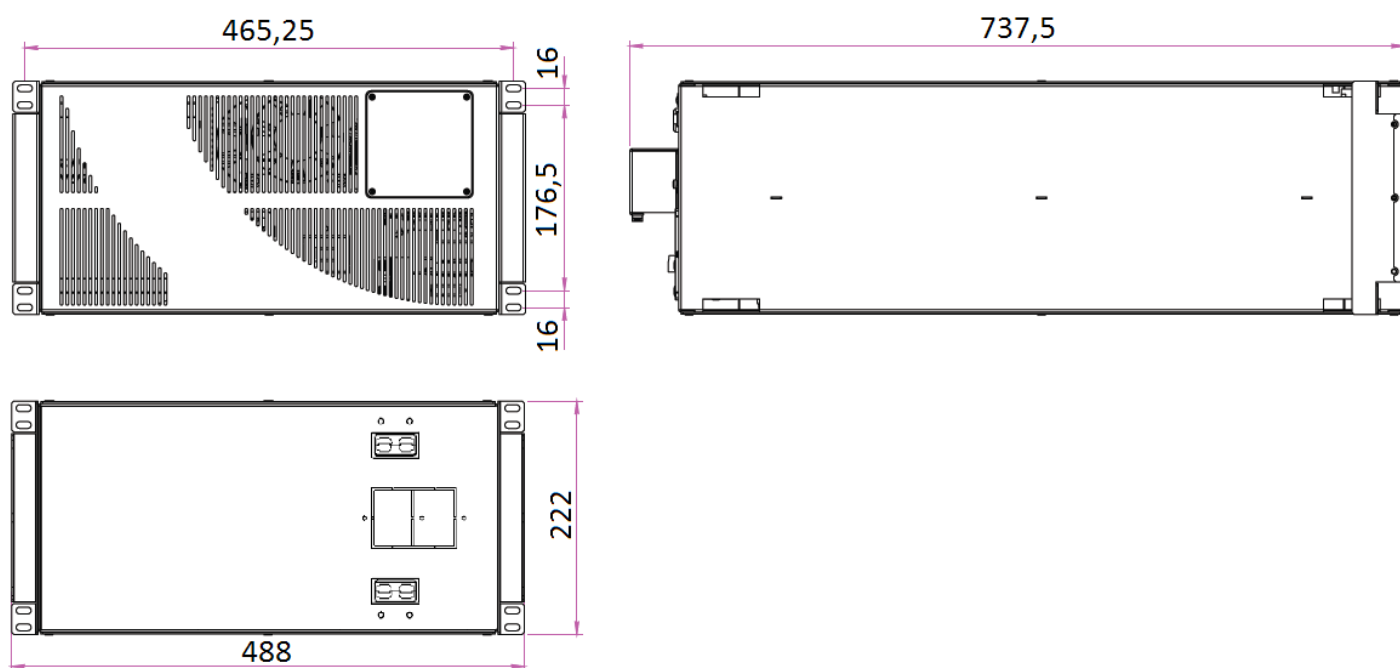
Рисунок 4. Внешний вид батарейного блока серии Solo MD (установка в стойку)
