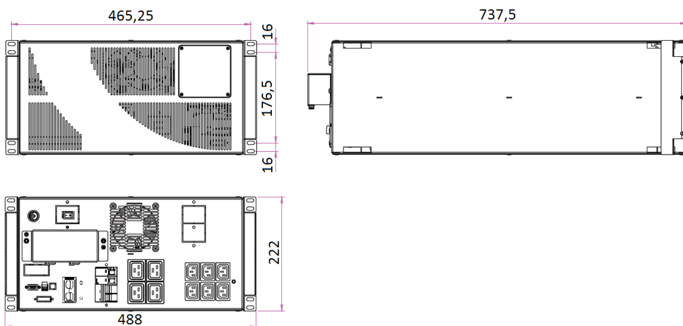
Рисунок 2. Внешний вид ИБП серии Solo MD (установка в стойку)
