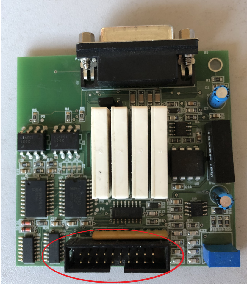
Рисунок 15. Плата AS400
