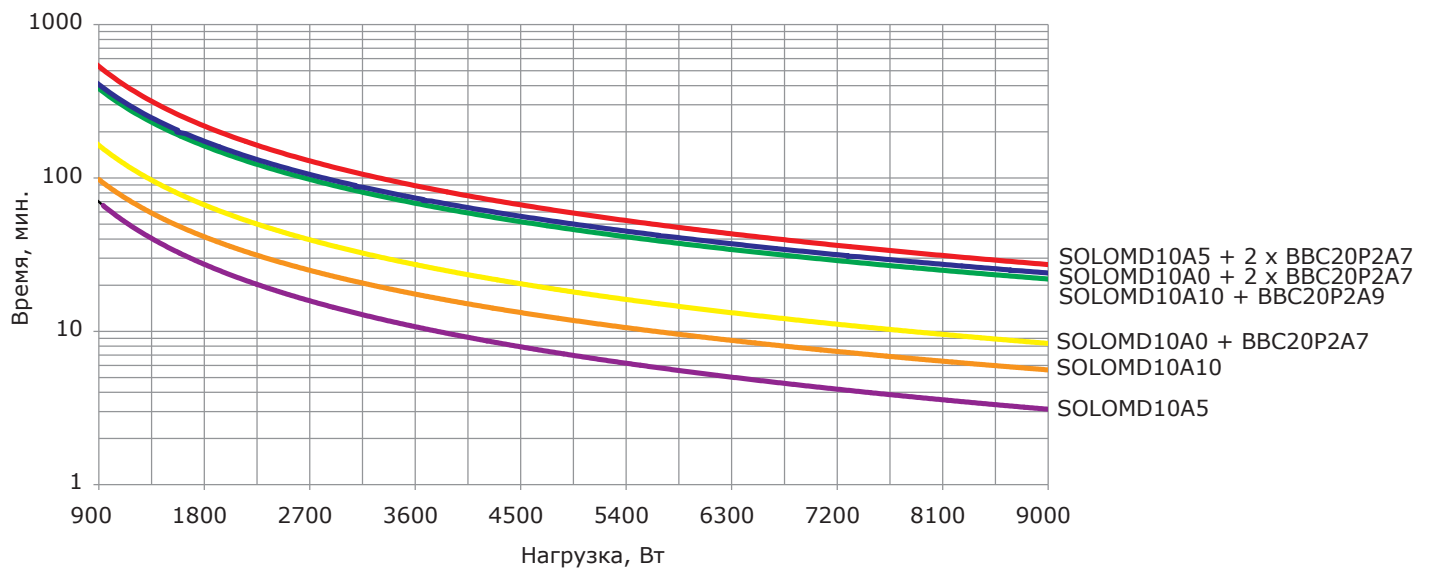
Рисунок 8 – Разрядные характеристики модели SOLOMD10
