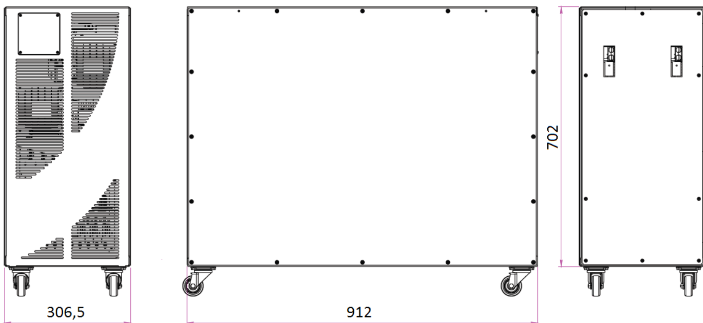
Рисунок 6. Внешний вид батарейного блока серии Solo MMB
