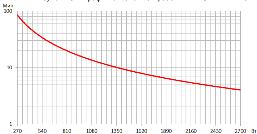
Рисунок 16 – График автономной работы ИБП SMALLT3A5
