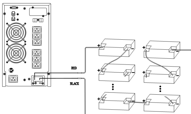
Рисунок 4 – Схема подключения внешних батарей.
