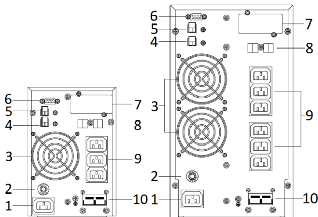
Рисунок 3 – Задняя панель ИБП SMALLT1 и SMALLT2 / SMALLT3
