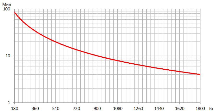
Рисунок 14 – График автономной работы ИБП SMALLT2A5
