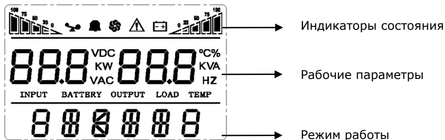
Рисунок 9 – Отображение параметров на экране ИБП
