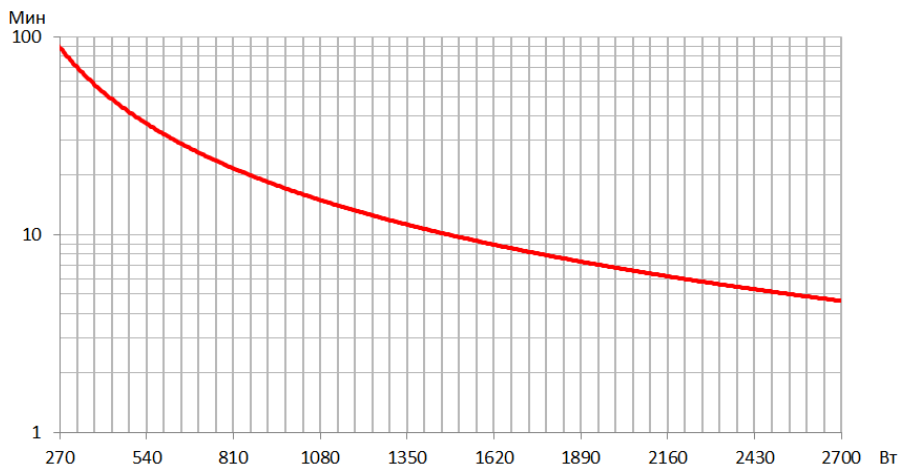
Рисунок 17 – График автономной работы ИБП SMALLT3A10
