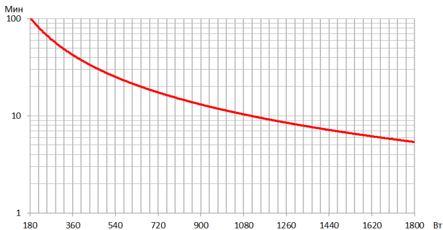
Рисунок 15 – График автономной работы ИБП SMALLT2A10
