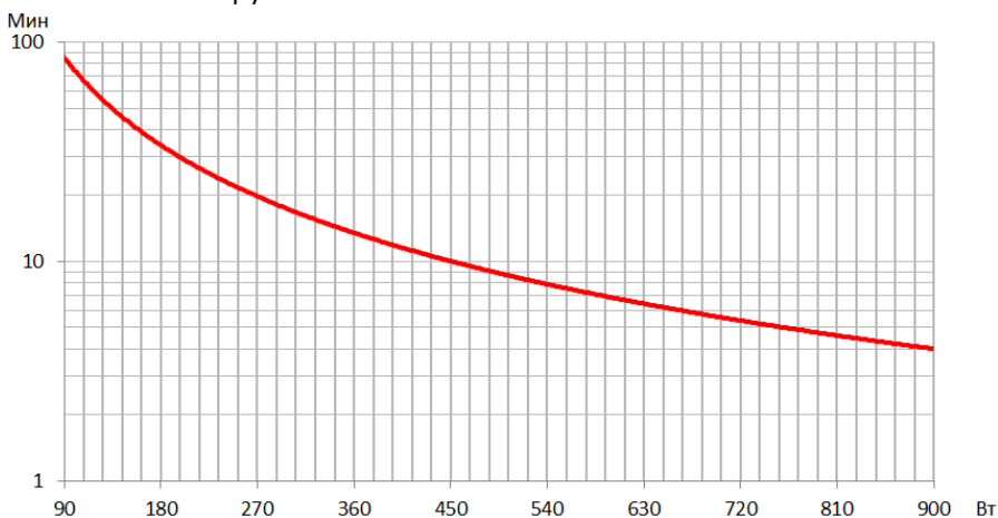
Рисунок 12 – График автономной работы ИБП SMALLT1A5
