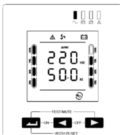
Рисунок 8 - Экран с кнопками управления ИБП
