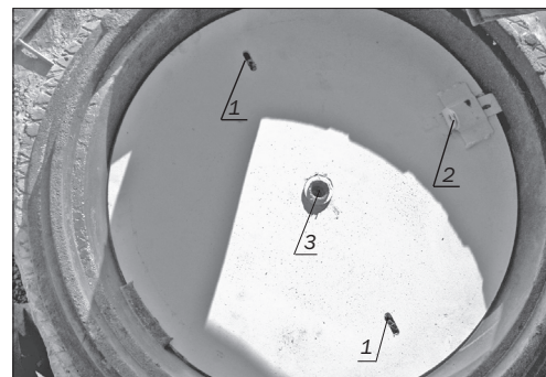
Рисунок 4.2 – Установленная нижняя крышка УЗЛ-Л (УЗЛ-Т): 1 – пазы нижней крышки; 2 – задвижка; 3 – гайка нижней крышки
