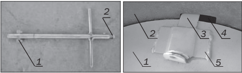
Рисунок 1.2 – Ключ ККЛ исполнения 0-9 1 - пластина; 2 - толкатель
